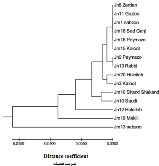
شکل ۵- آنالیز خوشه‌ای ۱۵ رقم نخل خرما با استفاده از روش UPGMA بر اساس نواحی توالی‌یابی شده ژن rbcL
