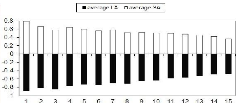
اکوتیپ ۱۰۱۲۶ / Ecotype 10126
