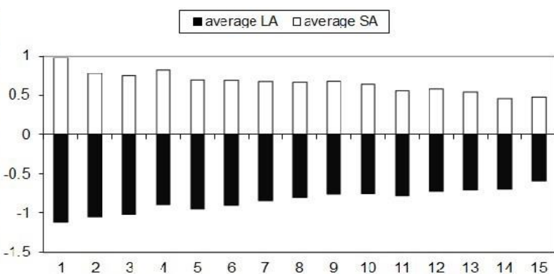
اکوتیپ ۱۴۲۸۷ / Ecotype 14287
