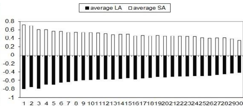
اکوتیپ ۱۴۲۴۵ / Ecotype 14245
